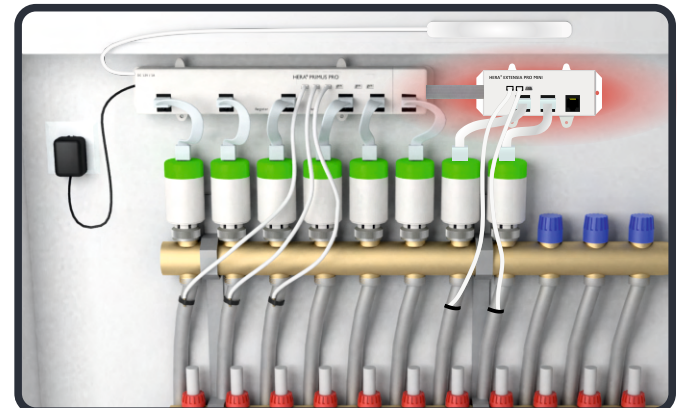
Funk-Fußbodenheizungs- leiste (Erweiterung)
