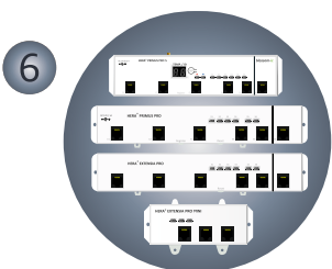
Hera+ Primus S/Primus/ Extensia/Mini PRO Funk-Fußbodenheizungsleiste zur Steuerung der Fußboden- heizung (6-Port-Modul / 3-Port-Modul)
