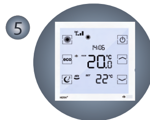
Hera+ Funk-Raumthermostat zur Steuerung der Fußbodenheizung in Verbindung mit den Funk- Fußbodenheizungsleisten
